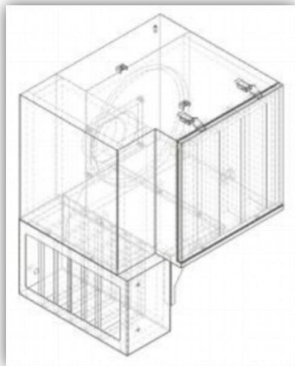
进气消音箱
